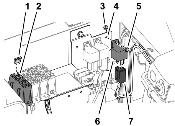
그림 36 2016년부터 생산된 장비
